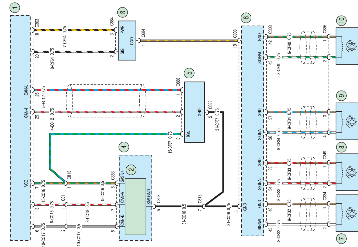
Схема 86. Антиблокировочная система (ABS) и система динамической стабилизации (ESP): 1, 6 – блок управления динамической стабилизацией (ESP); 2 – датчик положения рулевого колеса; 3 – датчик первичного давления в тормозной системе; 4 – спиральная пружина; 5 – датчик рыскания; 7, 8 – датчики частоты вращения передних колес; 9, 10 – датчики частоты вращения задних колес
