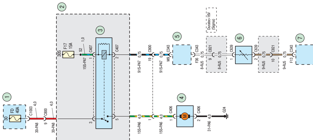
Схема 6а. Система охлаждения: 1 – монтажный блок предохранителей в моторном отсеке; 2 – монтажный блок предохранителей и реле за вешевым ящиком; 3 – реле вентилятора системы охлаждения двигателя; 4 – электродвигатель вентилятора системы охлаждения двигателя; 5, 7 – электронный блок управления двигателя; 6 – датчик температуры системы охлаждения двигателя
