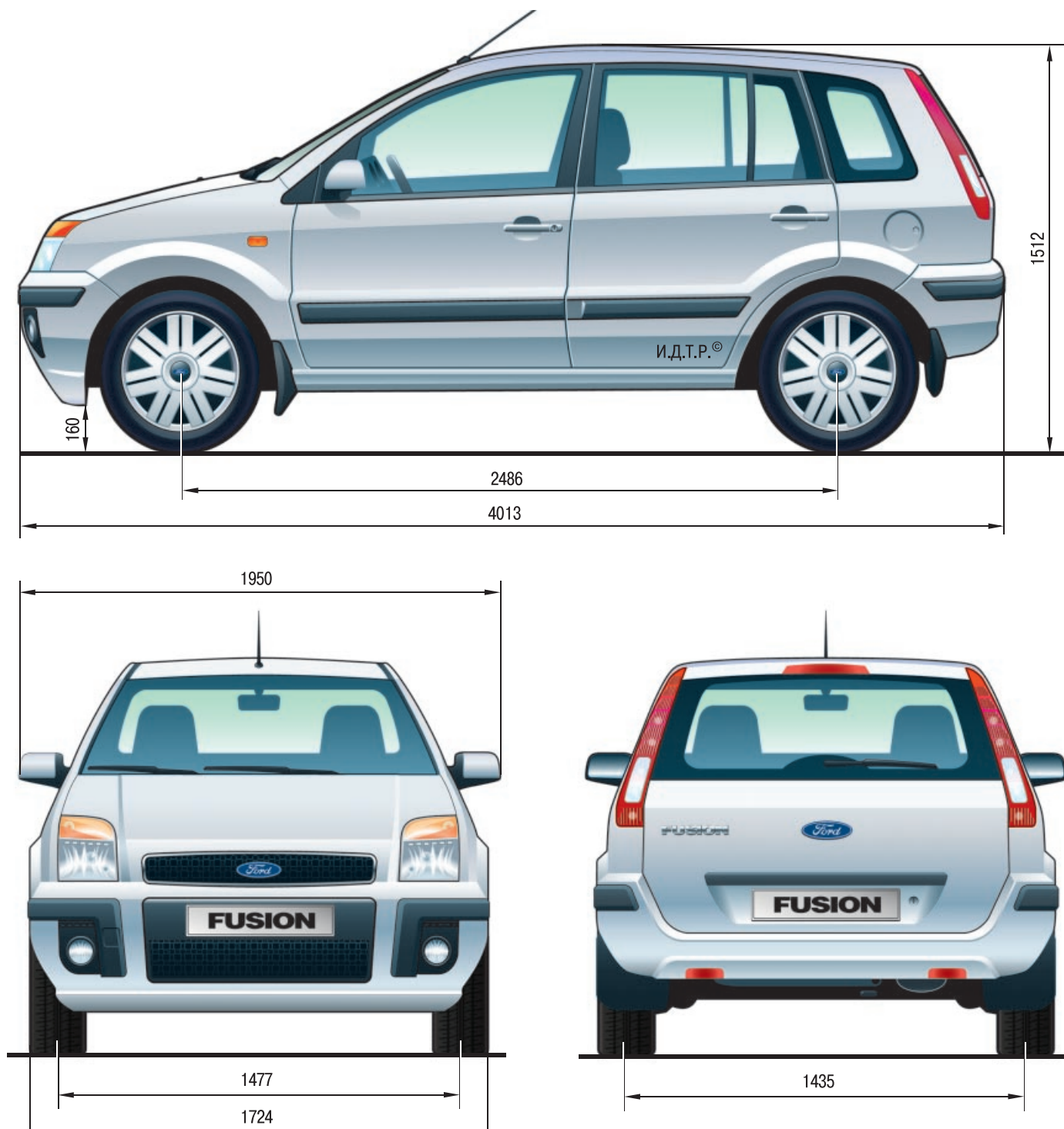
Рис. 1.3. Габаритные размеры автомобиля Ford Fusion
