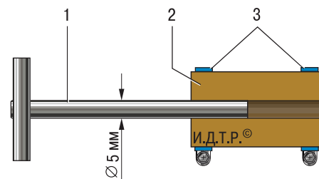
Рис. 5.29. Приспособление для притирки клапанов: 1 – металлический стержень; 2 – резиновый шланг; 3 – винтовые хомуты
