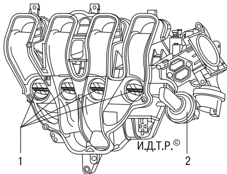
Рис. 5.6. Заслонки управления каналами впускного коллектора двигателя Duratec-NE: 1 – заслонки управления каналами впускного коллектора; 2 – привод заслонок управления каналами впускного коллектора
