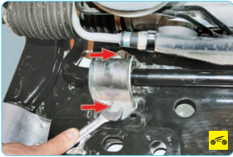
Рис. 7.3. Места установки подушек стабилизатора
