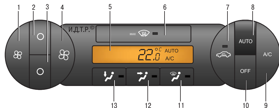
Рис. 1.12. Панель управления системой климат-контроля
