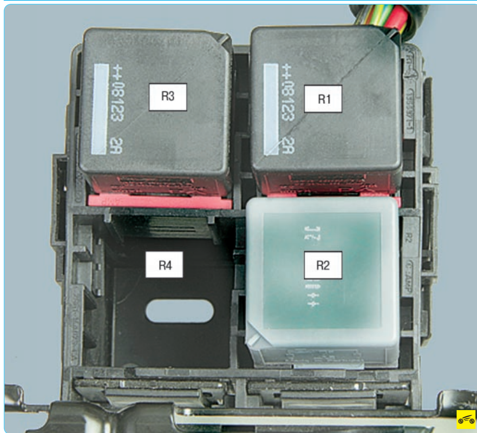
Рис. 10.3. Расположение реле в монтажном блоке, расположенном в подкапотном пространстве
