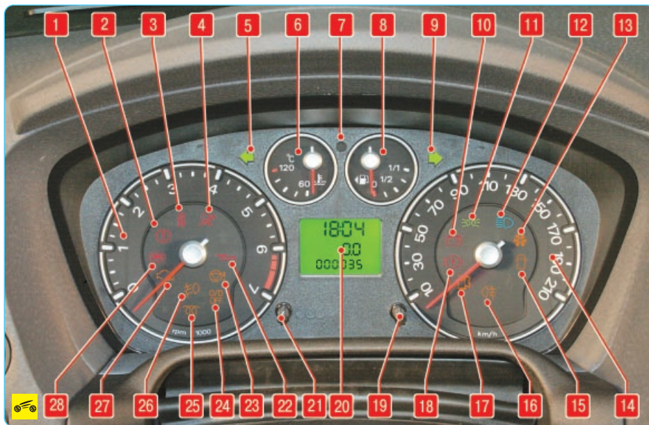
Рис. 1.9. Комбинация приборов
