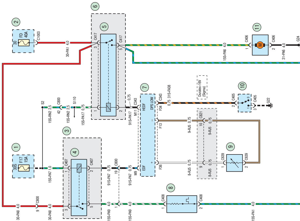
Схема 66. Система охлаждения: 1, 3 – монтажный блок предохранителей и реле за вешевым ящиком; 2 – монтажный блок предохранителей в моторном отсеке; 4 – реле вентилятора системы охлаждения двигателя; 5 – реле вентилятора системы охлаждения двигателя (высокая скорость); 6 – блок реле в подкапотном пространстве; 7 – электронный блок управления двигателем; 8 – резистор электровентилятора системы охлаждения двигателя; 9 – датчик температуры системы охлаждения двигателя; 10 – датчик высокого давления компрессора кондиционера; 11 – электродвигатель вентилятора системы охлаждения двигателя
