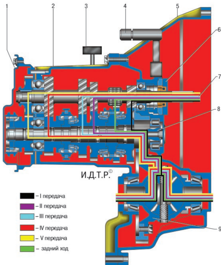
Рис. 6.3. Принципиальная схема пятиступенчатой механической коробки передач: 1 – задняя крышка картера коробки передач; 2 – картер коробки передач; 3 – салун; 4 – рабочий цилиндр гидропривода выключения сцепления; 5 – картер сцепления; 6 – подшипник выключения сцепления; 7 – первичный вал; 8 – вторичный вал; 9 – главная передача и дифференциал
