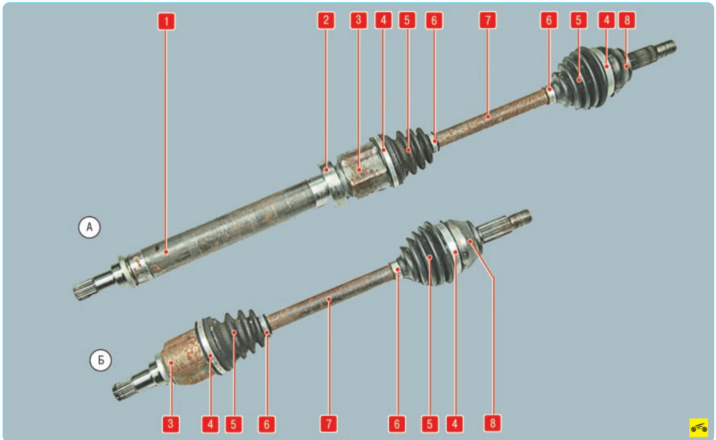
Рис. 6.7. Приводы передних колес: А – привод правого переднего колеса; Б – привод левого переднего колеса; 1 – промежуточный вал; 2 – подшипник промежуточной опоры; 3 – внутренние шарниры равных угловых скоростей; 4 – большие хомуты крепления чехлов шарниров; 5 – чехлы шарниров; 6 – малые хомуты крепления чехлов шарниров; 7 – вала приводов; 8 – наружные шарниры равных угловых скоростей
